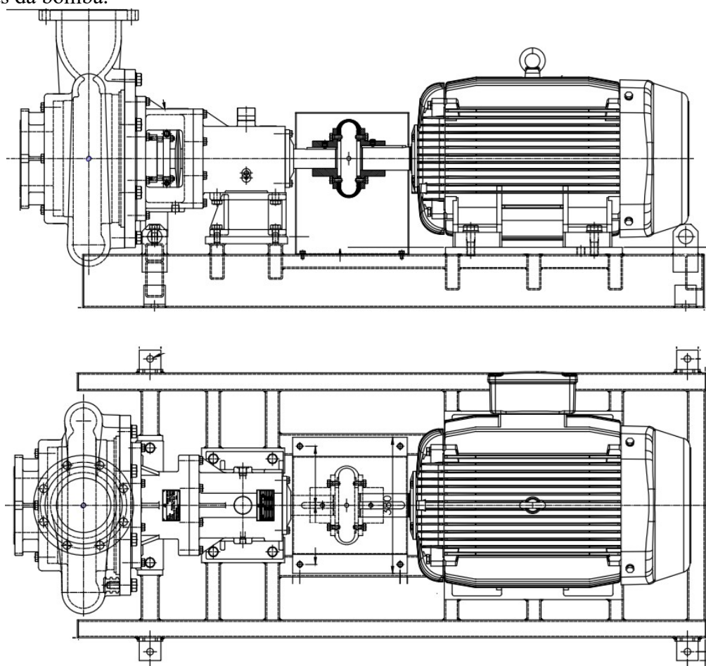
Figura 17 – Imagem do projeto construtivo de uma bomba centrífuga de Rotor Aberto série STAR OPEN da JAGUAR CI.
