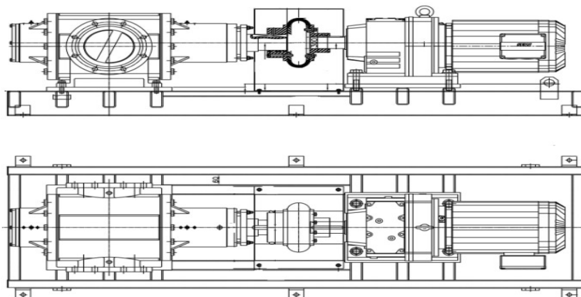
Figura 17 – Imagem do projeto construtivo de uma bomba mecânica JPP série WHITE BULL da JAGUAR CI, mancalizada com buchas.
