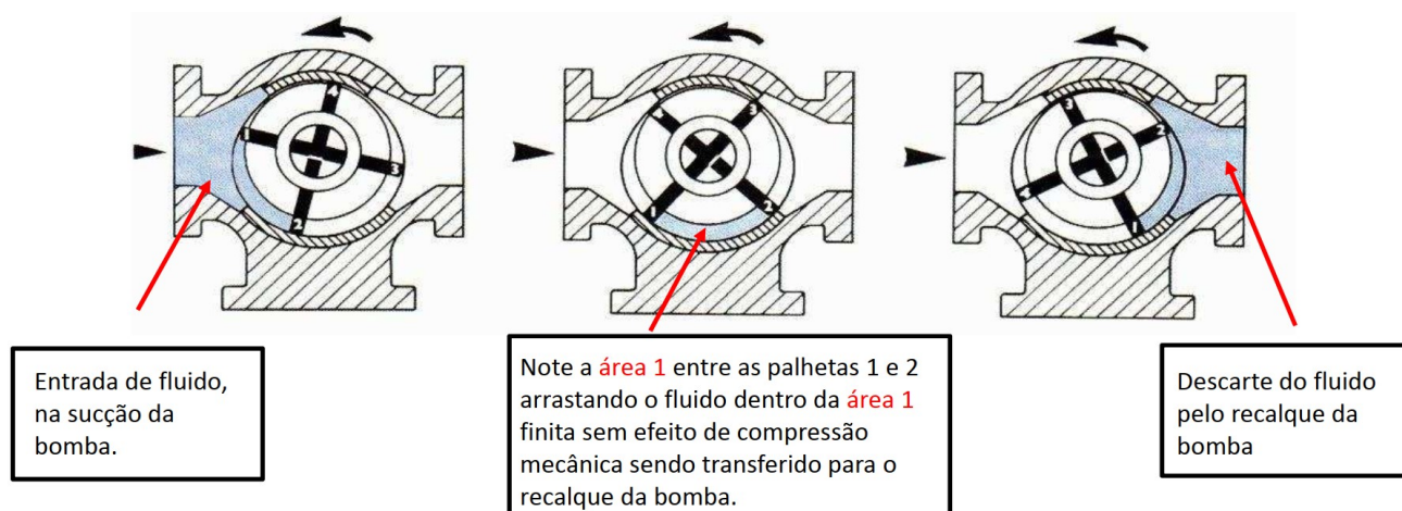
Figura 16 – Caracterização do transporte de fluidos no interior de uma bomba de deslocamento positivo de Palhetas.
