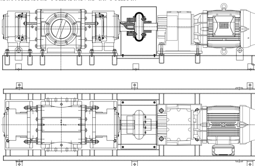
Figura 18 – Imagem do projeto construtivo de uma bomba mecânica JPP-ROL série WHITE BULL da JAGUAR CI.
