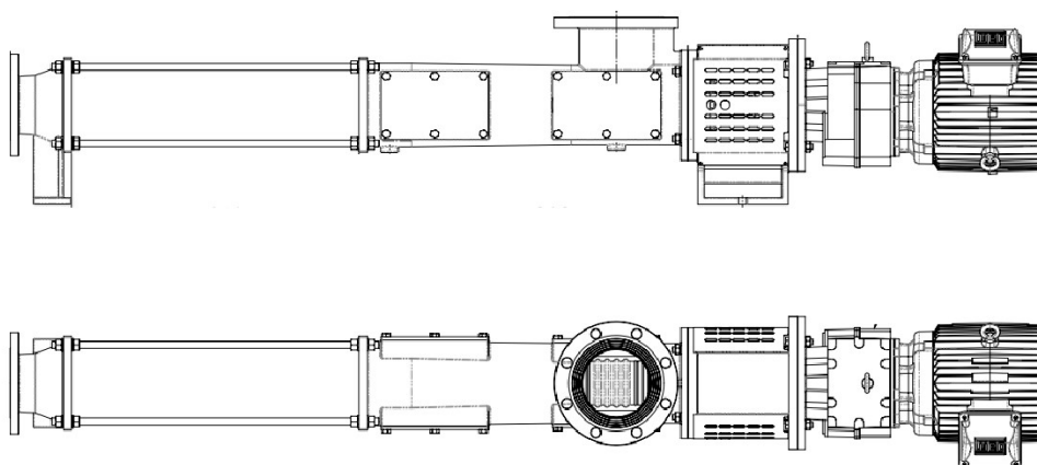
Figura 17 – Imagem do projeto construtivo de uma bomba helicoidais série SIMPLY CLEVER da JAGUAR CI.
